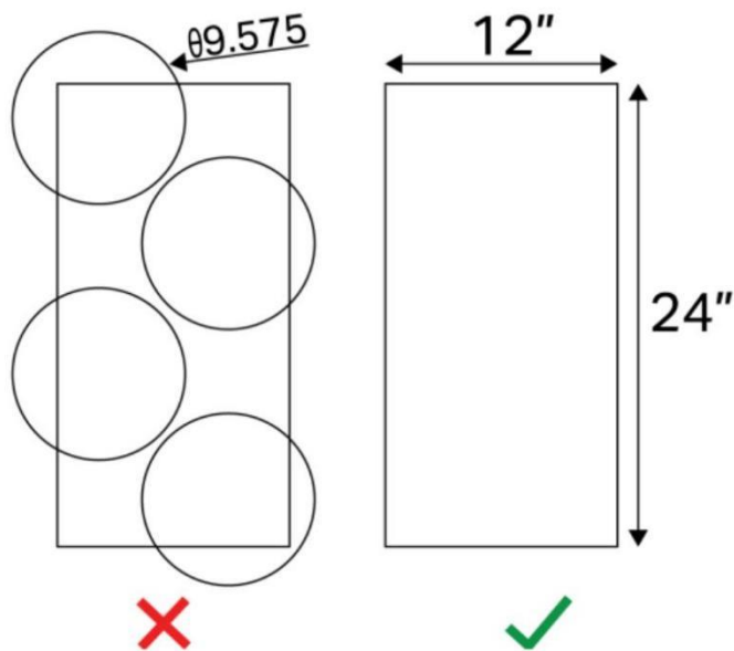
图 23 自制塑料件须可容纳于单块 12" x24" 的塑料板内
